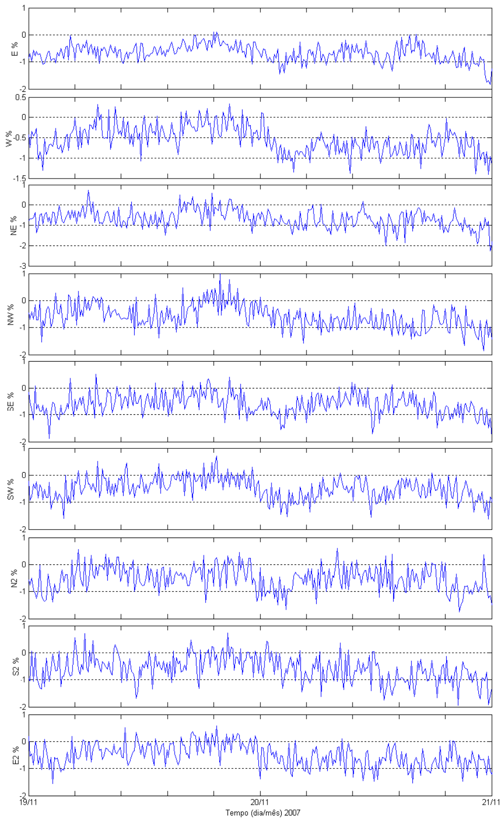
Figura 36 – De cima para baixo contagem de muons na direção leste, oeste, nordeste, noroeste, sudeste, sudoeste, norte 2, sul 2 e leste 2.
