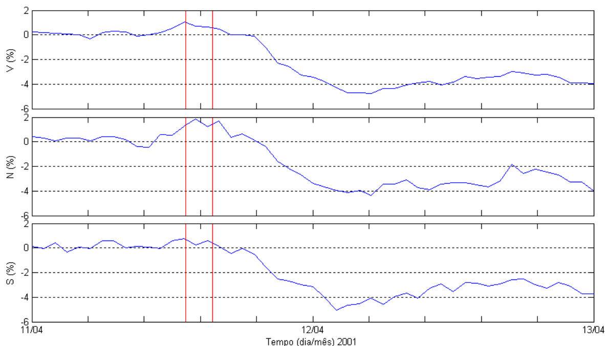
Figura 2 – De cima para baixo as contagens da variação percentual de muons na direção vertical, norte e sul.
