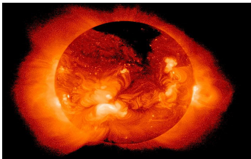
Figura 8 – A região escura no pólo do sol é um buraco coronal visto pelo telescópio de raios x do satélite Yohkoh. O Vento Solar que flui para fora é rápido. Não há emissão de raios x na região. Fonte: http://solarscience.msfc.nasa.gov/feature3.shtml
