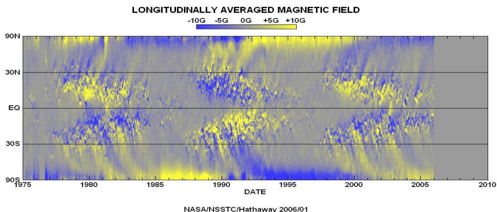
Figura 5 – Diagrama da Borboleta. É possível ver o ciclo solar através das cores em azul e amarelo pares de manchas. As manchas nascem em altas latitudes e migram para o equador. Campo magnético medido em Gauss. FONTE: http://www.nasa.gov/vision/universe/solarsystem/solar_cycle_graphics.html
