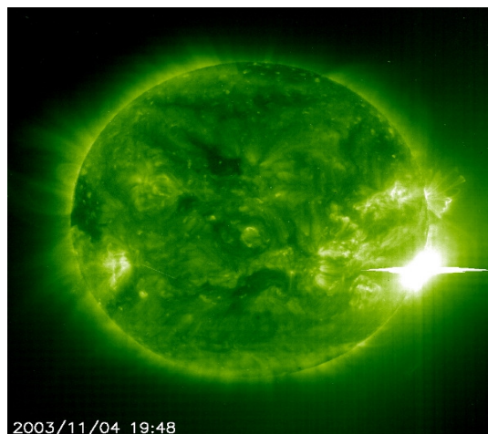
Figura 10 – A explosão solar (“flare”) na figura é o ponto mais brilhante da imagem. Obtida pelo instrumento EIT em 04 de novembro de 2003, a bordo do satélite SOHO, em 195 Å.
