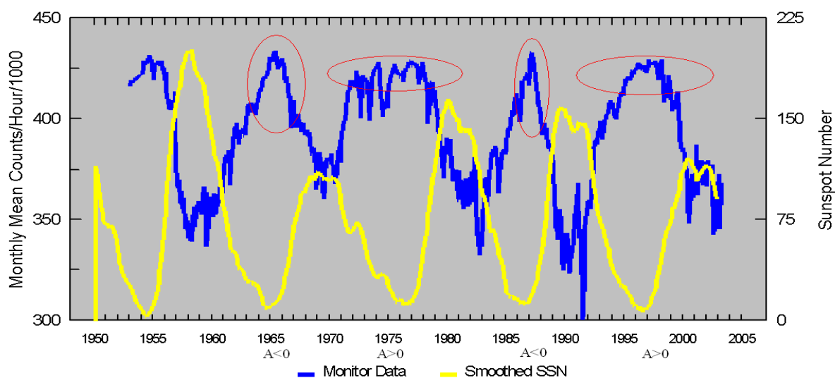
Figura 7 – Em azul dados obtidos pelo monitor de nêutrons – Climax da Universidade de Chicago. Em amarelo dados de manchas solares. Os círculos vermelhos mostram a variação de 22 anos. FONTE: http://www.ngdc.noaa.gov/stp/SOLAR/COSMIC_RAYS/image/cr_ssn.gif
