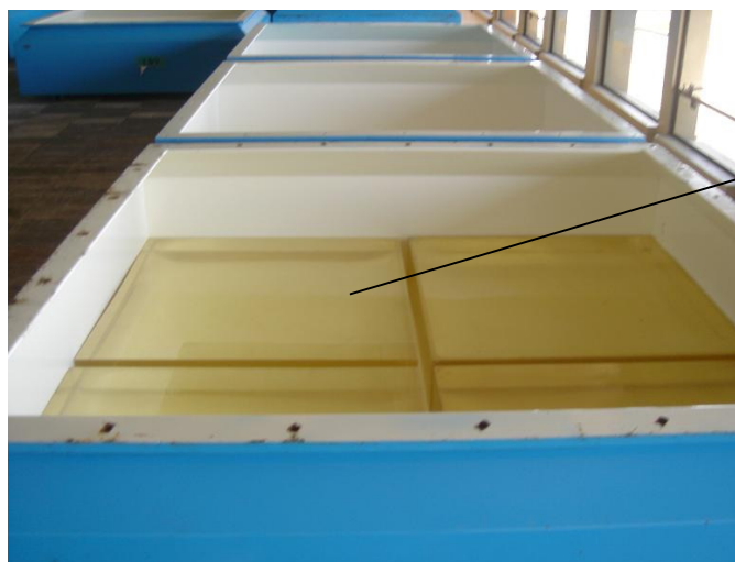
Figura 19 – Quatro cintiladores lado a lado formando uma área de superfície de 1m 2 . Os cintiladores estão colocados em caixa de metal com espessura de 1,6 mm.
