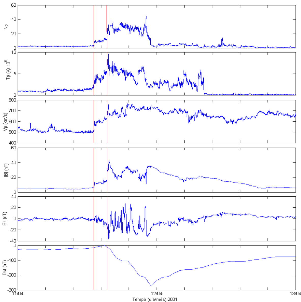
Figura 1 – De cima para baixo densidade, temperatura, velocidade do vento solar, modulo do campo magnético, componente z do campo magnético e índice geomagnético Dst.
