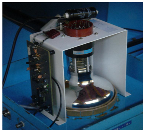
Figura 32: Fotomultiplicadora
